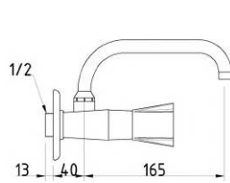
BASIN FAUCET WALL LAVABO BATARYASI DÖNER KUĞU BORU
