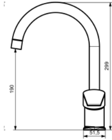
SINK MIXER LONG EVİYE BATARYASI UZUN DİK BORU
