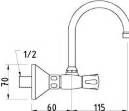
WASHBASIN FAUCET LAVABO BATARYASI DÖNER BORU
