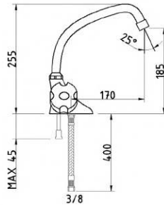
SINK FAUCET LONG EVYE BATARYASI UZUN KUĞU
